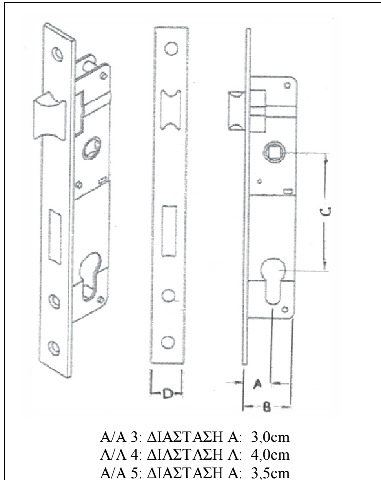
Σχέδιο 2. α/α 3, 4, 5: ΚΛΕΙΔΑΡΙΕΣ ΑΛΟΥΜΙΝΙΟΥ ΑΣΦΑΛΕΙΑΣ
