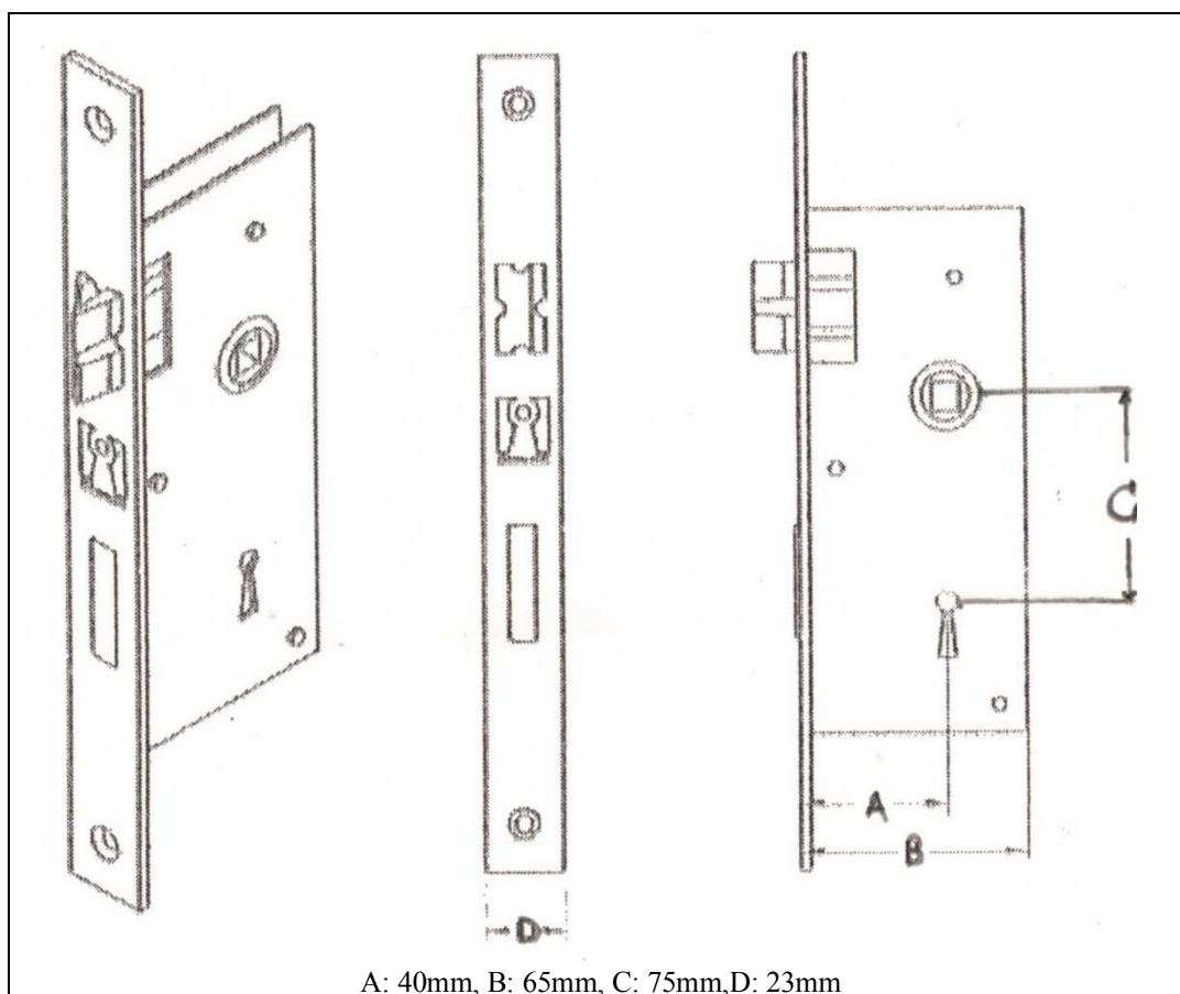
Σχέδιο 1. α/α 1: ΚΛΕΙΔΑΡΙΕΣ ΜΕΣΟΠΟΡΤΑΣ (ΔΑΚΛΔ00010)
